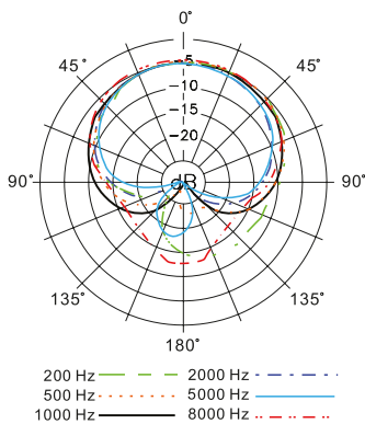
Диаграмма направленности
