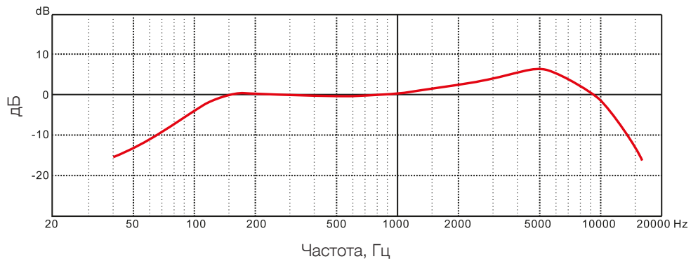
Частотный диапазон
