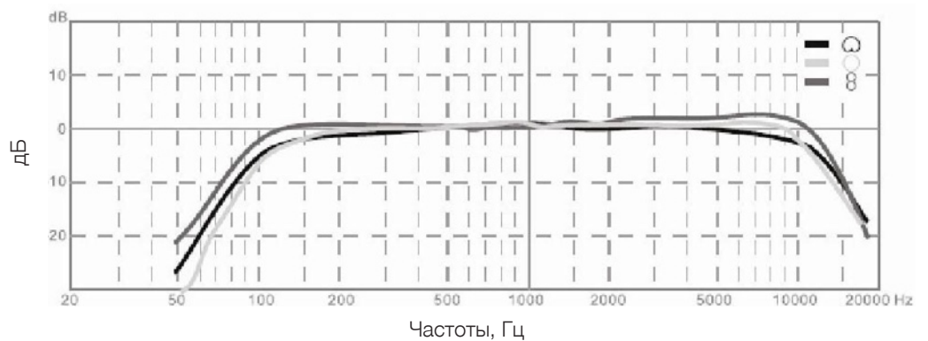
Частотный диапазон
