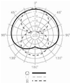
Диаграмма направленности
